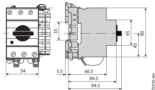
Автоматический выключатель для защиты электродвигателей MS325
