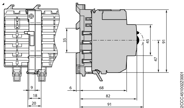
Разъединитель нейтрали
